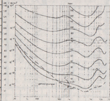
— — — — — Oeff. v. de gehoordrempel vgt. Fletcher-Munson (1933) — — — — — Oeff. v. de gehoordrempel vgt. Robinson en Scharf (1955) — — — — — Lijnen van gelijke luidheid (isofonen) volgens Robinson en Scharf
