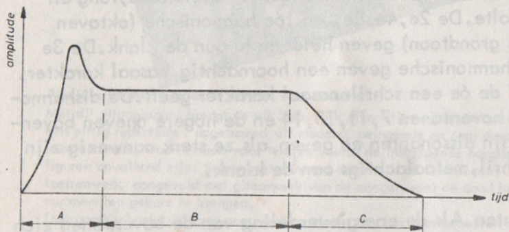
A = inslingerverschijnsel B = periodieke trillingstoestand C = uitslingerverschijnsel
